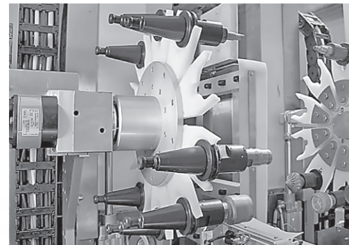
「T10」自動ツールチェンジャー
